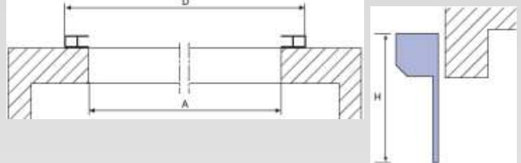
Linksroller außen auf Mauerwerk montiert
