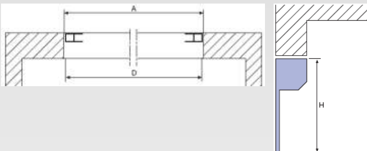
Rechtsroller zwischen der Laibung montiert
