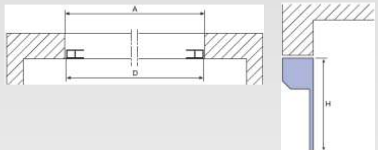
Linksroller zwischen der Laibung montiert
