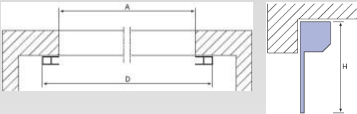
Rechtsroller hinter dem Anschlag montiert
